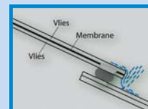
REGENBESTENDIGHEID
